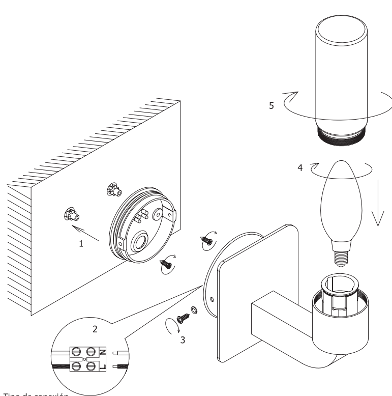
Tipo de conexión Type of connection B
